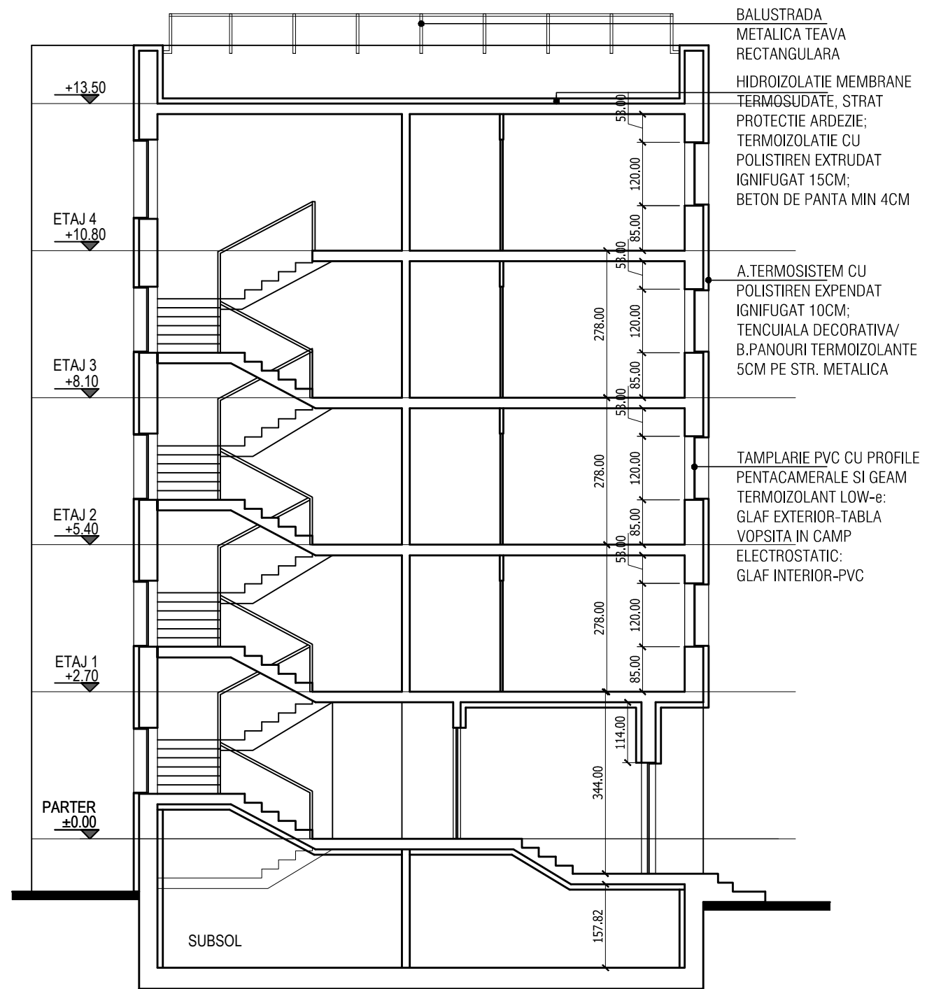
SECTIUNE TRANSVERSALA - PROPUS
