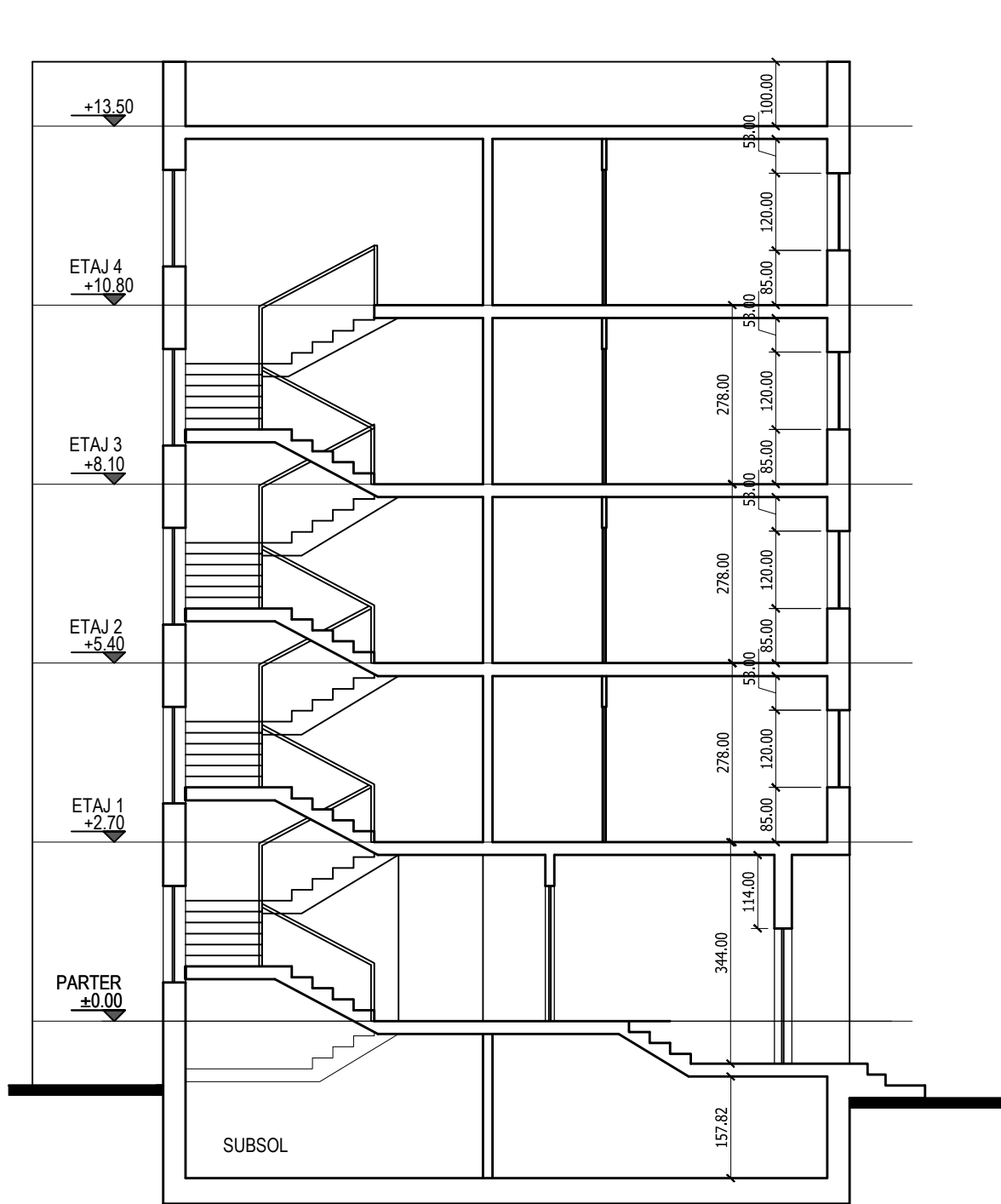
SECTIUNE TRANSVERSALA - EXISTENT
