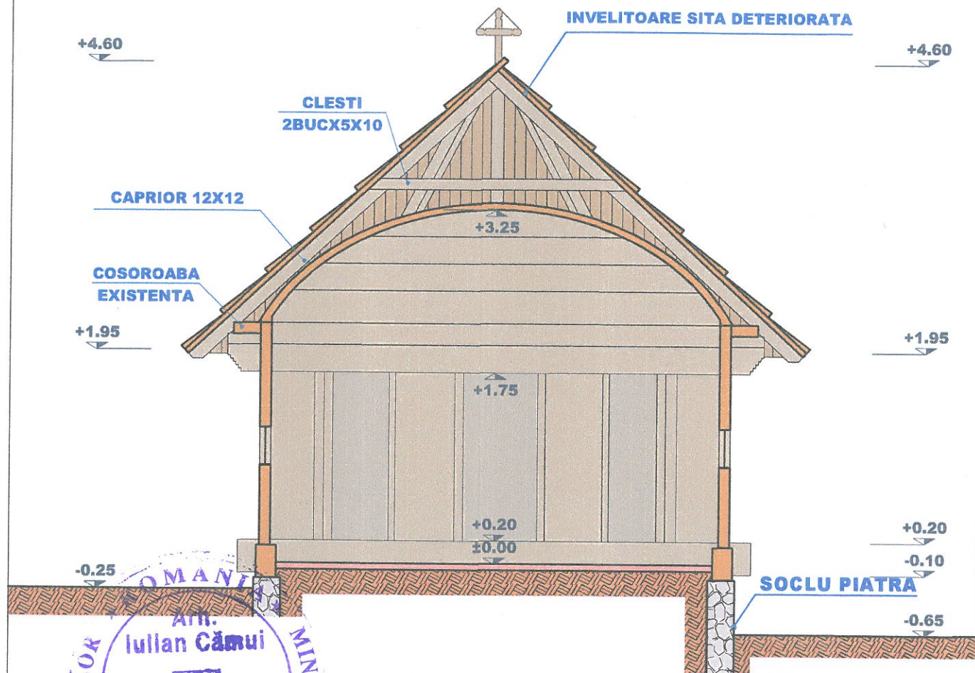
SECTIUNEA b-b scara 1:50
